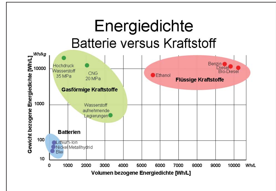
Bild 28: Vergleich der volumenbezogenen Energiedichten in Wattstunden pro Liter (Wh/L) von Batterien und Kraftstoffen; Quelle: Toyota
